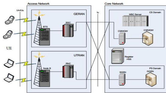
Gambar 5. Skema Struktur Jaringan HSDPA
