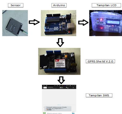
Gambar 8. Blok Diagram Sistem Pendeteksi Kebocoran
