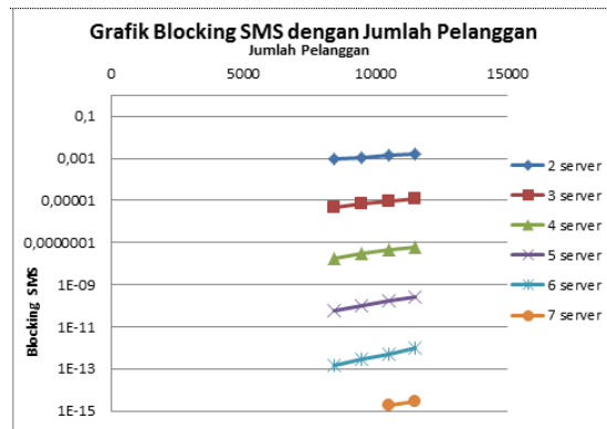
Gambar 12. Grafik Blocking SMS dengan Jumlah Pelanggan
