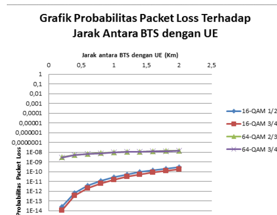
Gambar 13. Grafik Probability Packet Loss terhadap Jarak antara BTS dengan UE
