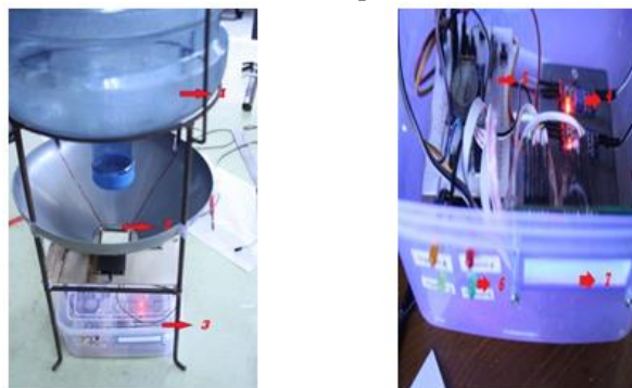
Gambar 9. Realisasi Tool Pendeteksi Kebocoran Data Informasi Yang Ditampilkan Pada LCD
